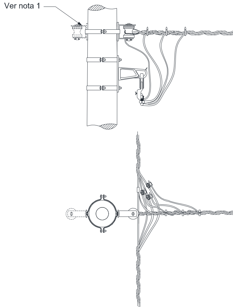
Figura 24 – Estruturas derivação tangente – S11 – S13 (alternativa)
